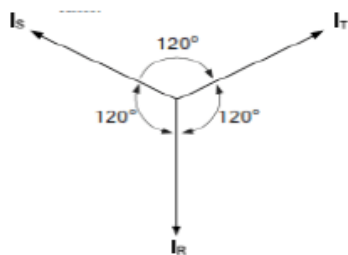
Gambar. Vektor Diagram Arus Seimbang
