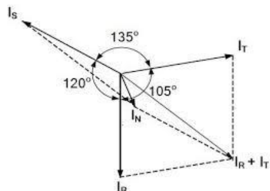
Gambar 2.11. Vektor Diagram Arus Tidak Seimbang
