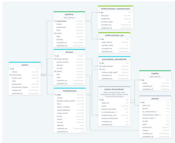
Gambar 3. ERD
