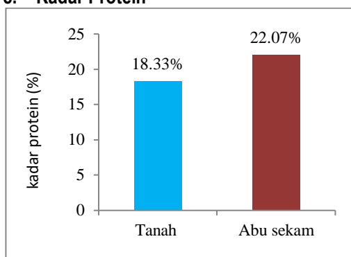
Gambar 4. Kadar Protein
