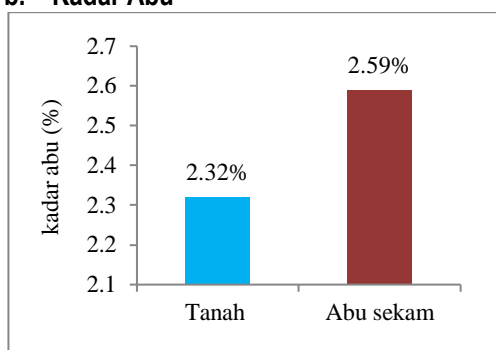
Gambar 3. Kadar Abu
