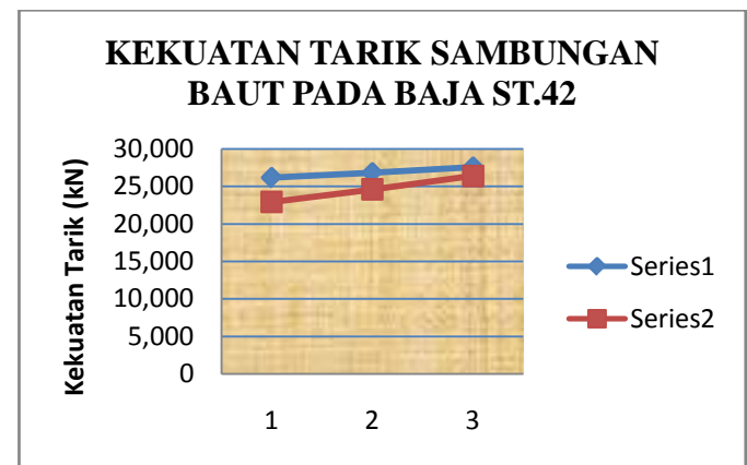
Gambar 2. Grafik Kekuatan Tarik Sambungan Baut
