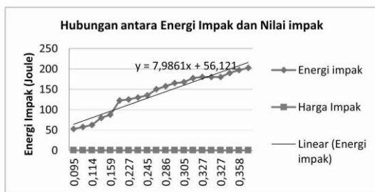
Gambar 2. Grafik Ketangguhan Hasil Pengelasan GMAW Pada Baja ST 42 dengan Pola Gerakan Zig-Zag Elektroda
