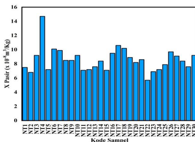
Gambar 4. Grafik Nilai Suseptibilitas Magnetik Pada Ke-30 Sampel Gumuk Pasir Sumalu.
