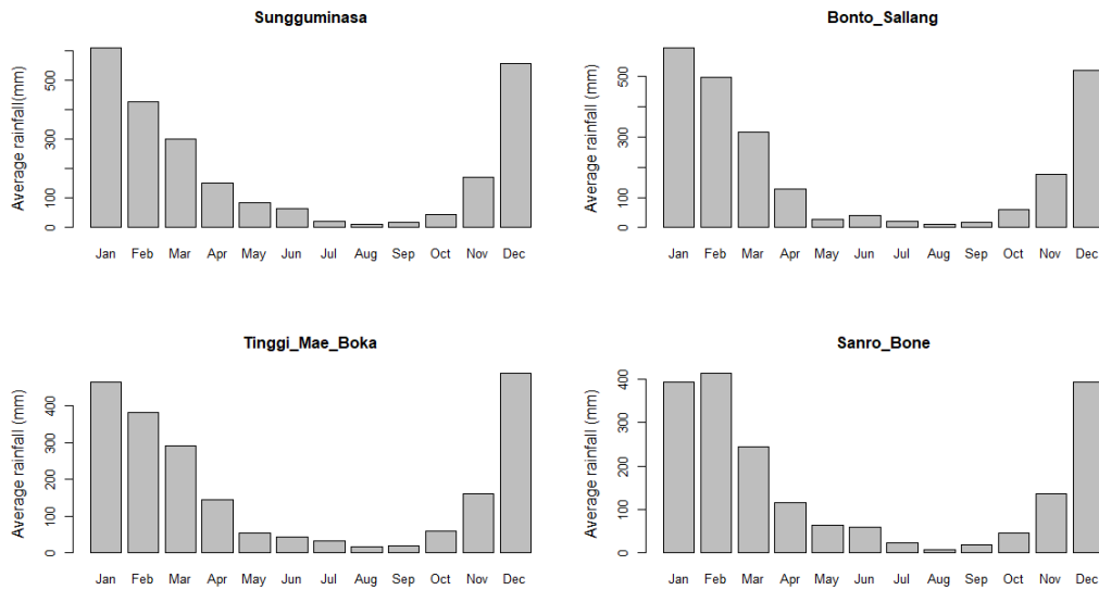
Gambar 2. Rata-rata hujan bulanan periode 1996-2020
