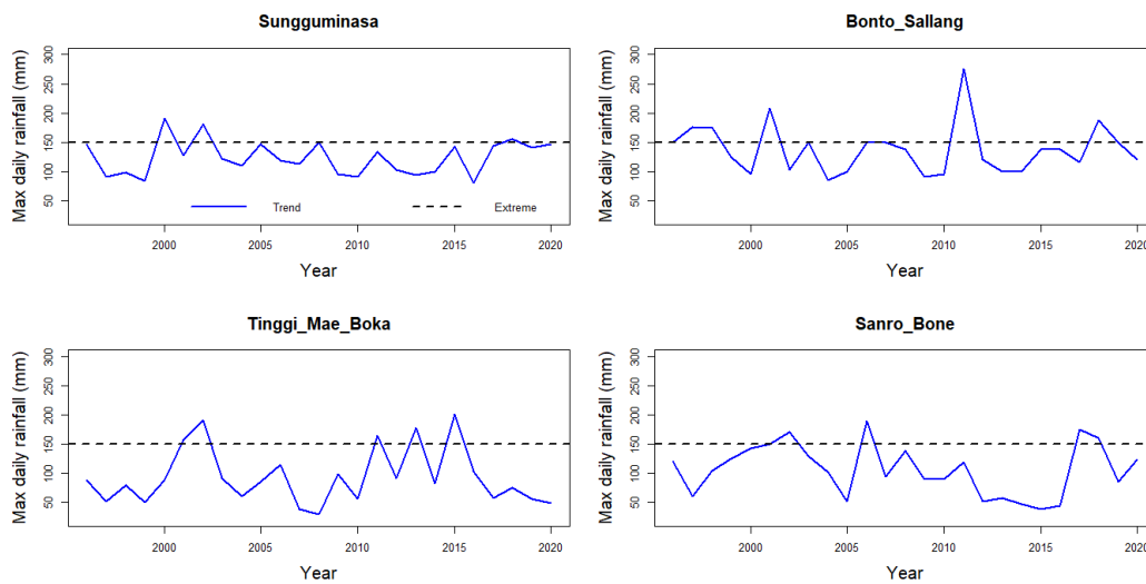
Gambar 3. Hujan harian maksimum tahunan periode 1996-2020
