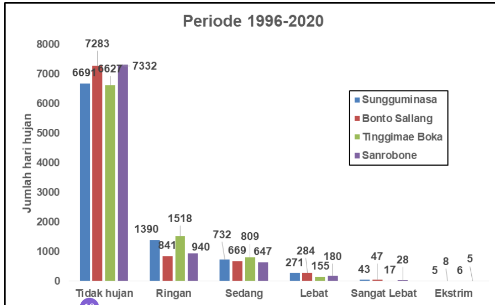
Gambar 1. Jumlah hari hujan berdasarkan kategori hujan harian
