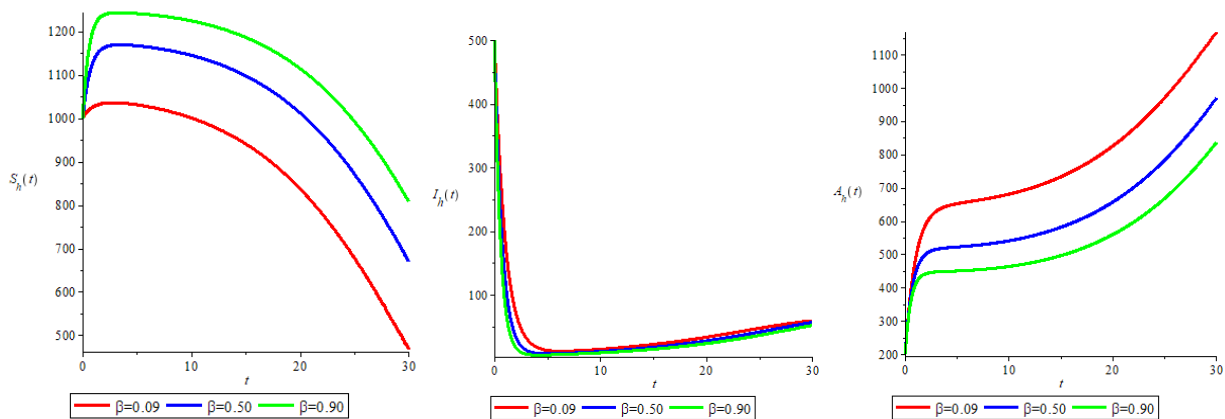
Gambar 2 Dinamika populasi manusia karena adanya pengobatan pada manusia
