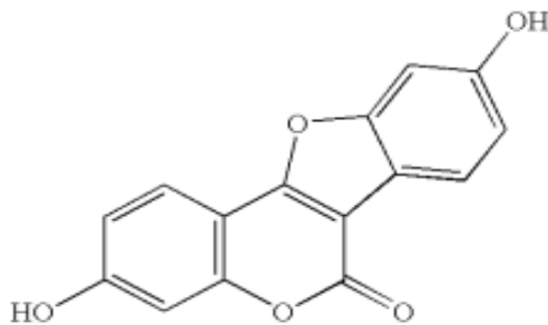
Gambar 8.4 Struktur Coumestrol
