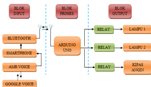
Gambar 2. Desain Perancangan Blok Antar Bagian
