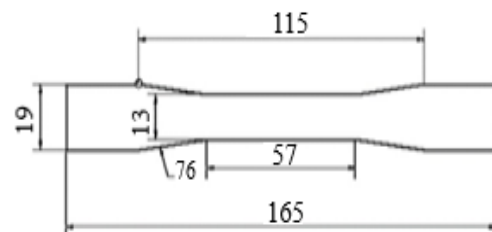
Gambar 5: Spesimen eksperimen uji tarik Data lengkap dari Gambar 5 di atas disajikan dalam Tabel-2 di bawah ini:
