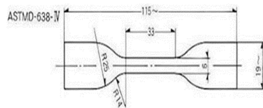
Gambar 4: Contoh Spesimen uji tarik
