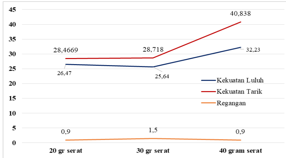
Gambar 6: Grafik hasil pengukuran uji tarik
