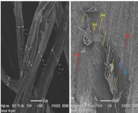
Gambar 13: Struktur Mikro Variasi Serat 40 gram
