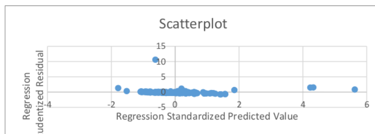
Gambar 3. Uji Heterokdasitas
