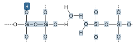
Gambar 5. Ikatan Hidrogen antar \equiv\text{Si-OH}
