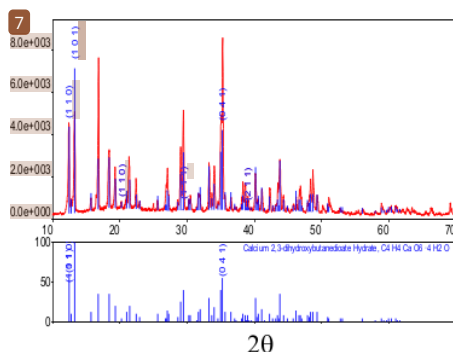
Gambar 6. Difraktogram Kristal CaTT Hasil Sintesis
