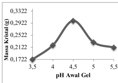
Gambar 2. Grafik Massa Kristal CaTT pada Variasi pH Gel Metasilikat
