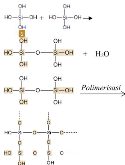
Gambar 4. Reaksi Polimerisasi Gel Metasilikat
