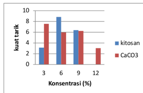
Gambar 4. Uji Kuat Tarik Bioplastik
