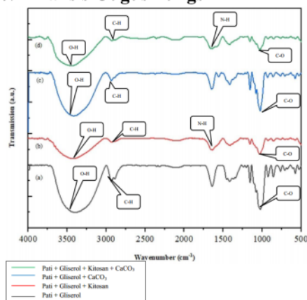
Gambar 7. Spektrum Analisis FTIR Bioplastik
