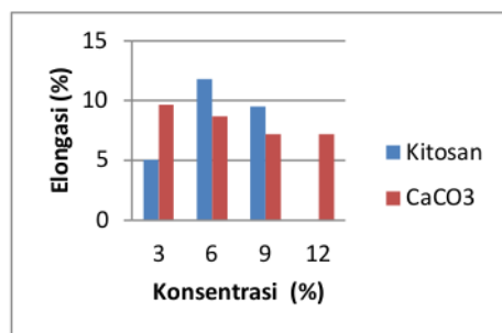
Gambar 5. Uji Elongasi Bioplastik
