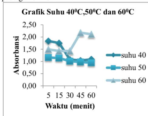
Gambar. 1 Grafik Pengaruh Waktu Pemanasan Terhadap Absorbansi
