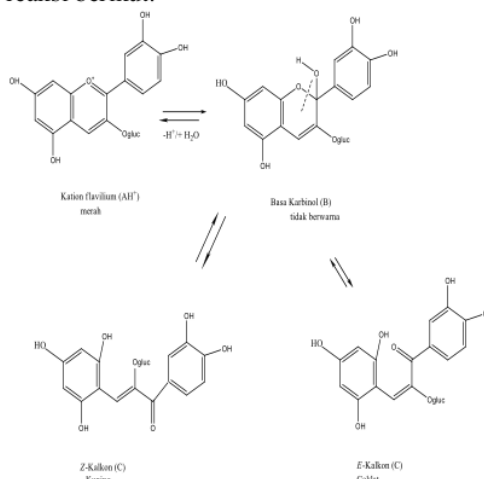
Gambar. 4.5 Gambar Dekomposisi Struktur Antosianin
