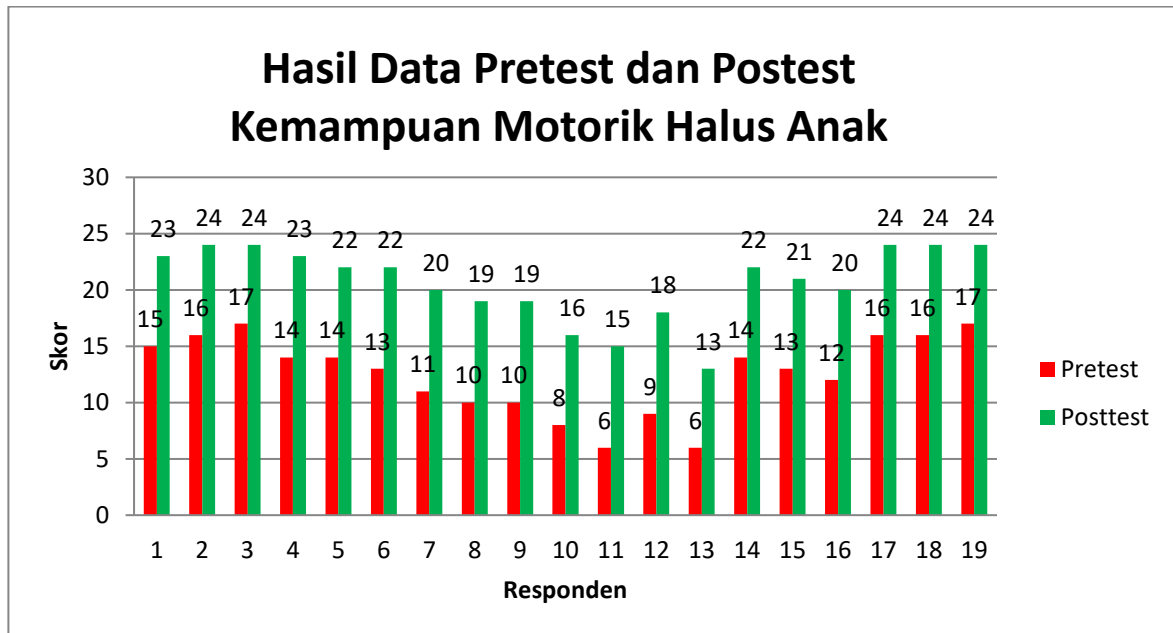
G.1 Histogram
