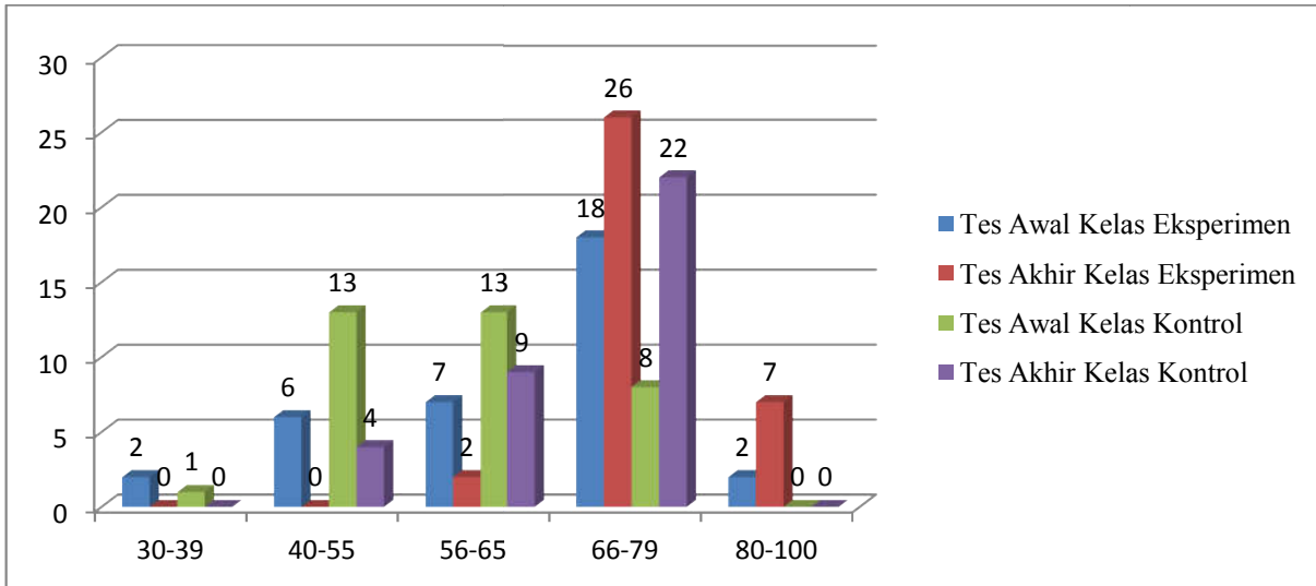
Gambar 1. Grafik rata-rata tes siswa
