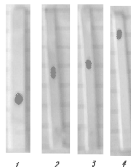
Gambar 1. Kromatogram KLT Isolat 1
