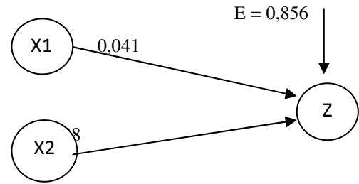
Gambar 4.7. Model hubungan langsung X1 dan X2 terhadap Z
