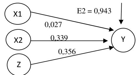
Gambar 4.8. Model hubungan langsung X1, X2 dan Z terhadap Y
