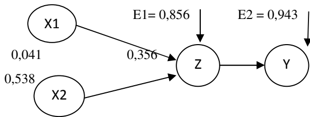
Gambar 4.9. Model hubungan tidak langsung X1, X2 dan Z terhadap Y
